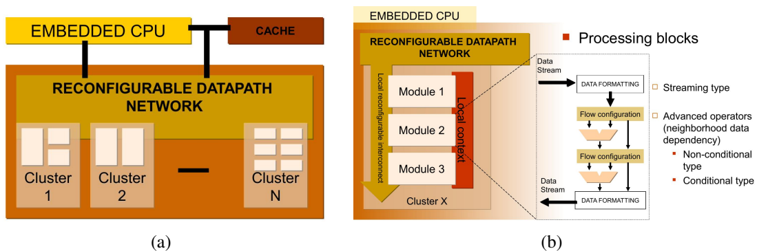
FIGURE 12.4 – Organisation interne du processeur reconfigurable CarVision.
