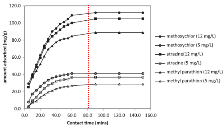
Figure III-3 : Représentation de cinétiques d'adsorption sur charbon actif (Gupta et al. 2011)
