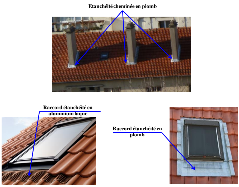
Figure 73 : Exemples de situations-typiques associées aux éléments d'étanchéité
