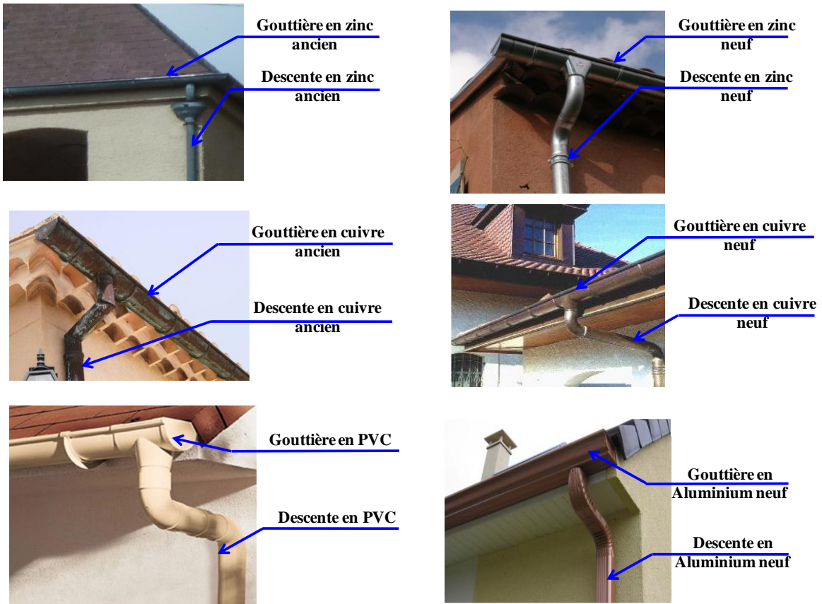
Figure 70 : Exemples de situations-typiques associées à la gouttière et la descente
