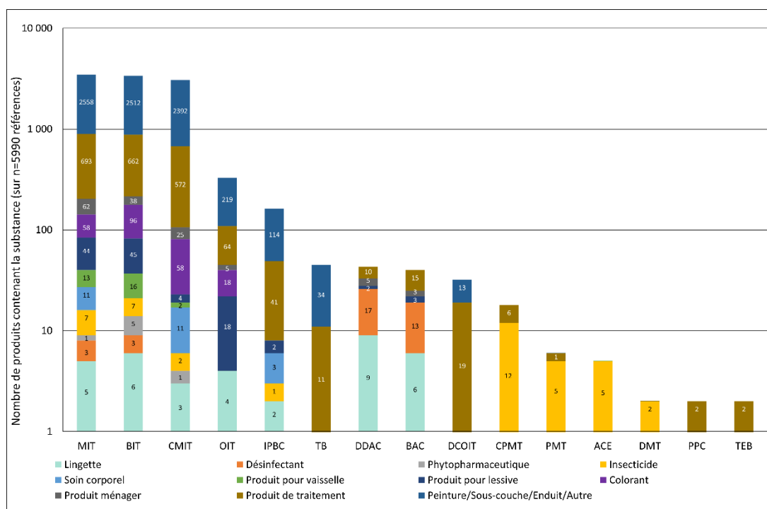
Figure 4. Nombre de produits recensés contenant les substances biocides d'intérêt sur n=5990 références (échelle logarithmique)
