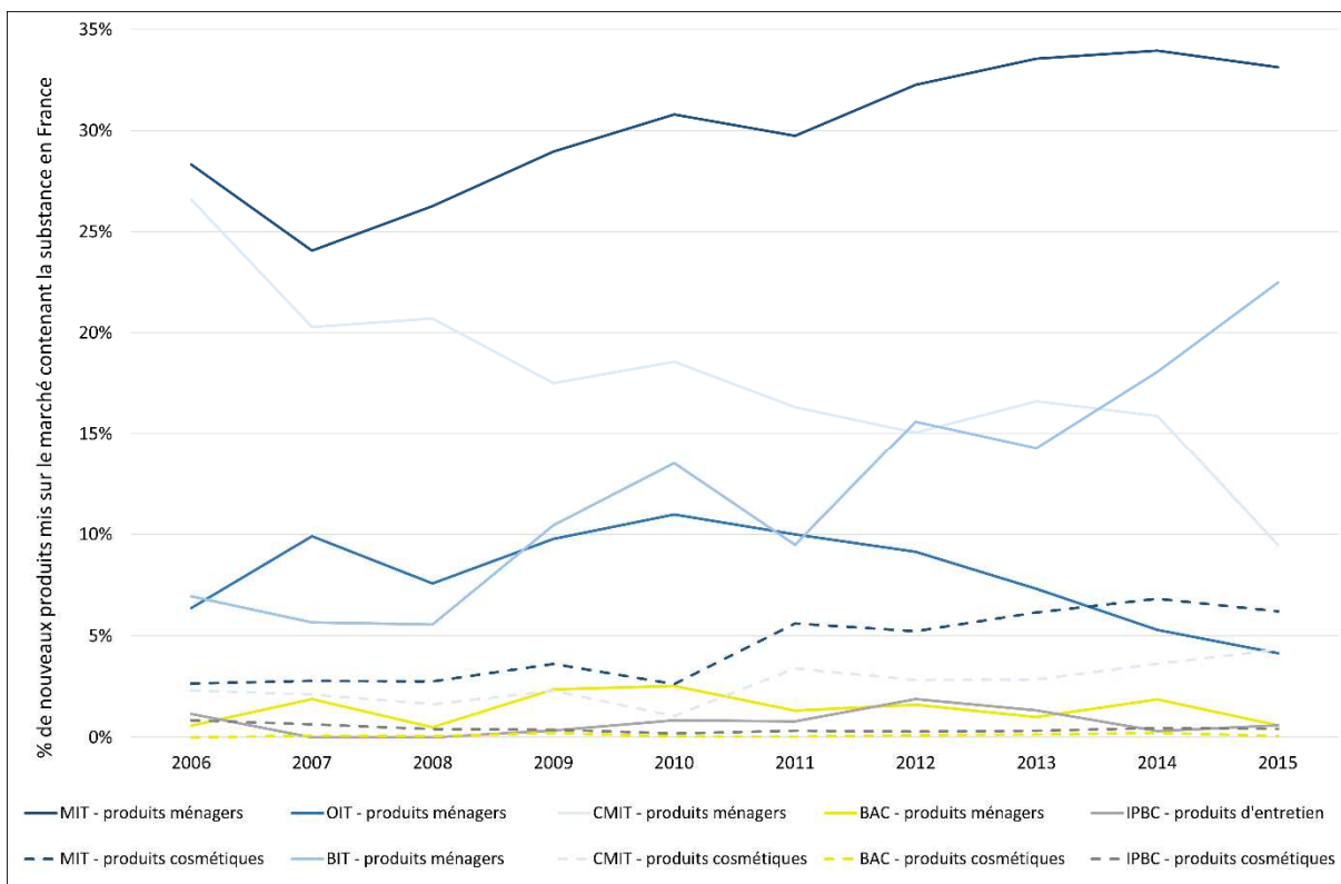
Figure 3. Évolution du pourcentage de nouveaux produits mis sur le marché qui contiennent les substances biocides sélectionnées dans le cas des produits ménagers (traits pleins) et des produits cosmétiques (pointillés) entre 2006 et 2015 (source Mintel)
