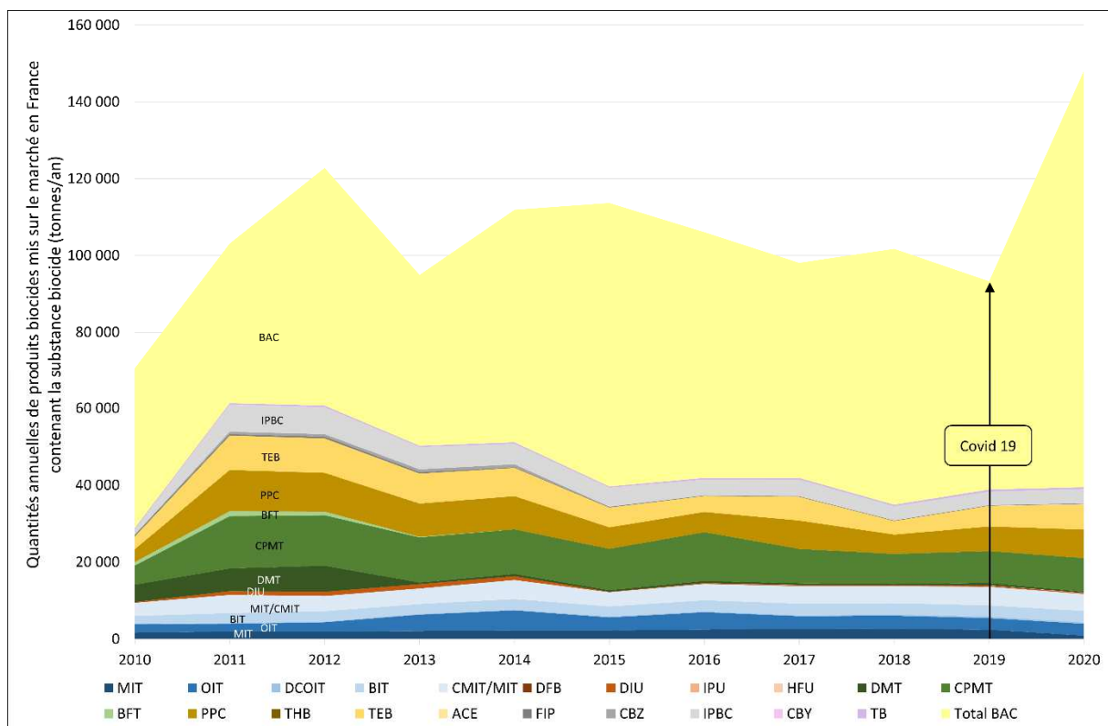
Figure 1. Évolution des quantités annuelles de produits biocides mis sur le marché en France et contenant la substance biocide entre 2010 et 2020 (source SIMMBAD)
