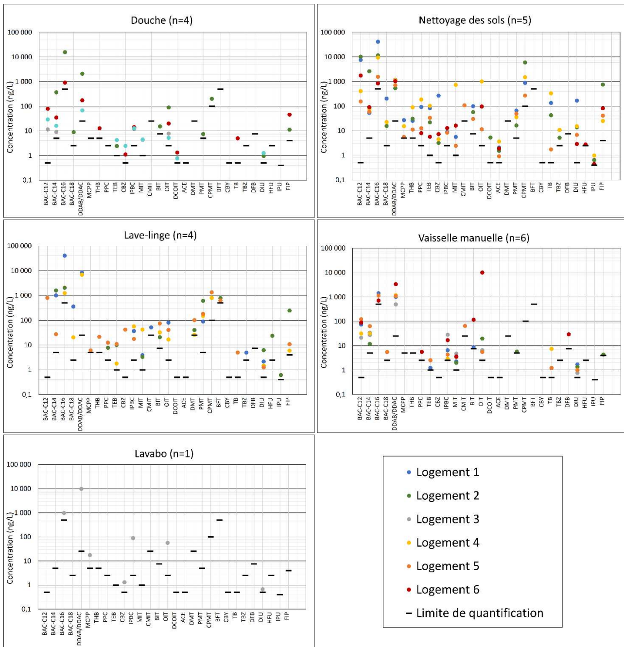
Figure 5. Concentrations (ng/L) en substances biocides dans les eaux grises pour chaque type d'eau grise, pour les sept logements échantillonnés (échelle logarithmique, les limites de quantification sont représentées avec des tirets noirs)
