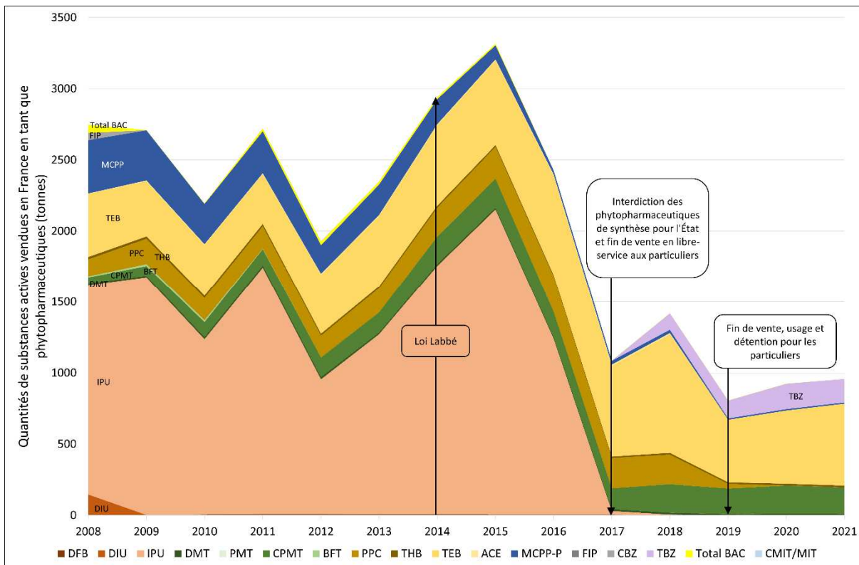
Figure 2. Évolution des quantités de substances actives de phytopharmaceutiques vendues en France entre 2008 et 2021 (source BNVD)
