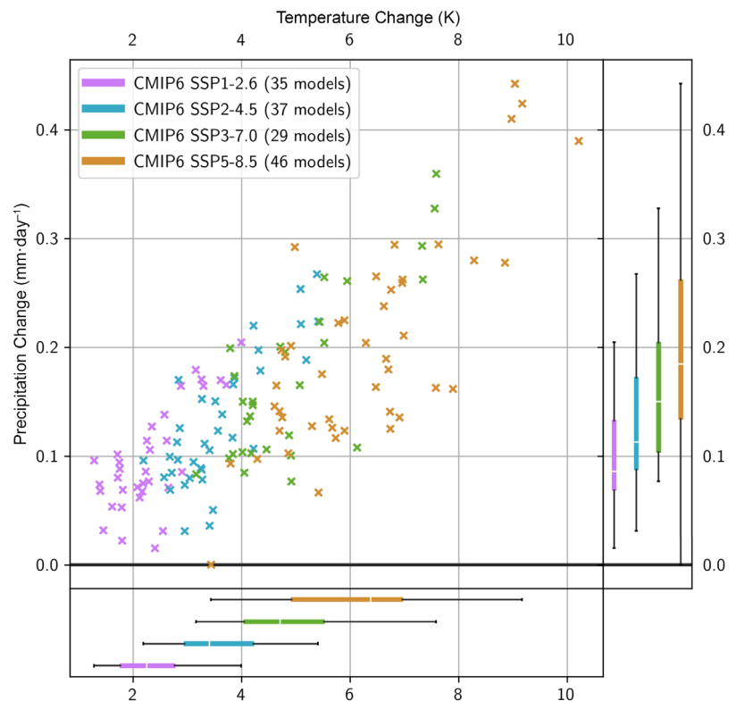
(b) CMIP6
