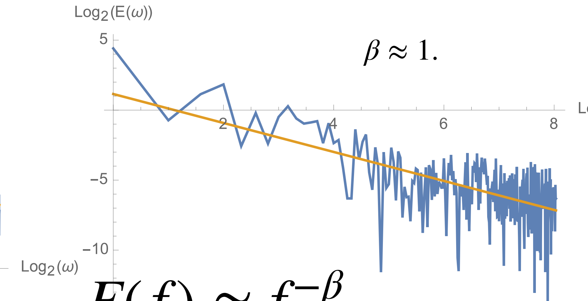
Vostok Dust
