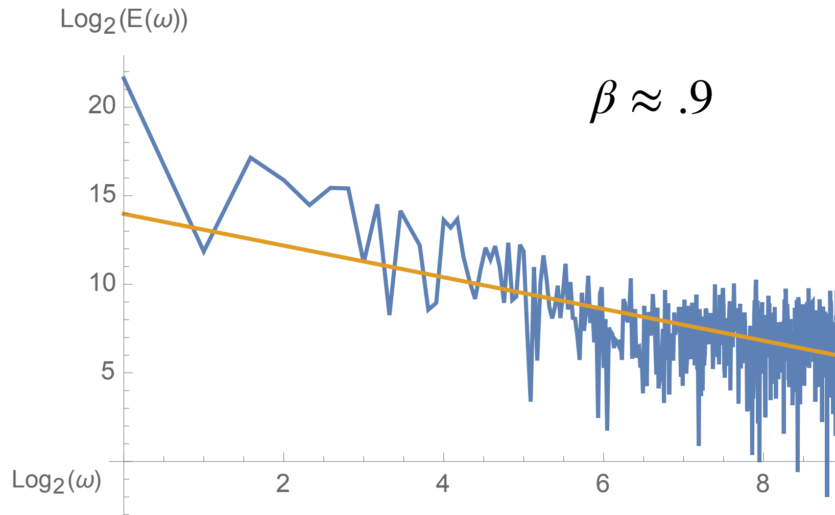
Vostok Na
