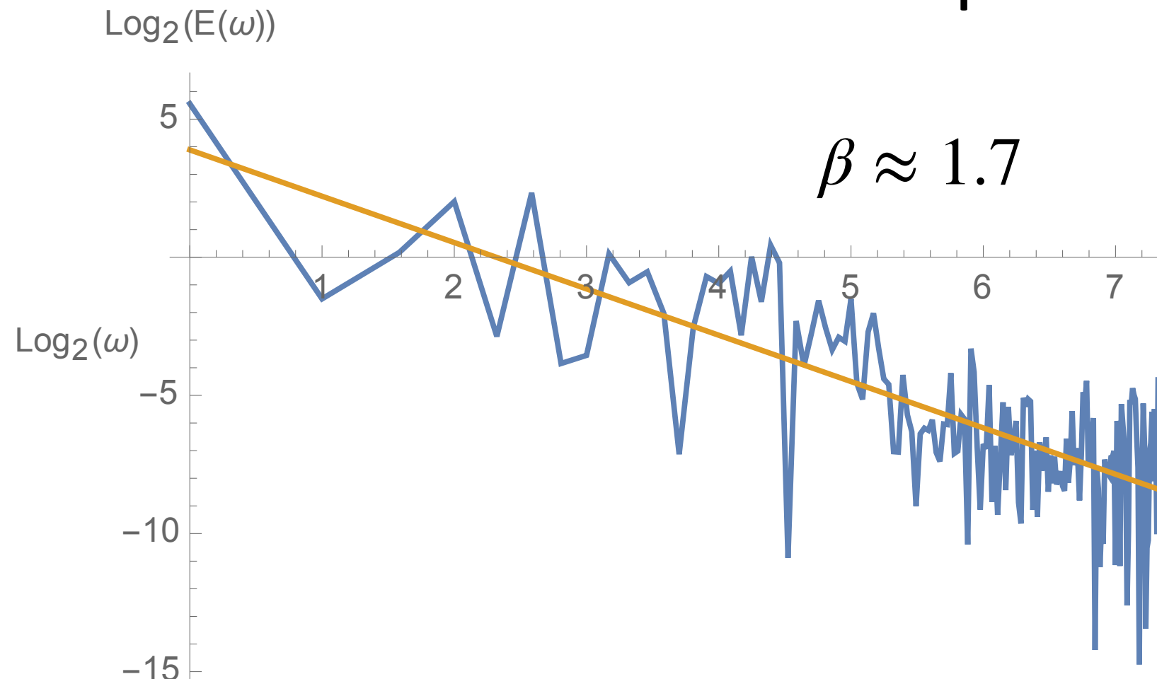
Vostok Na
