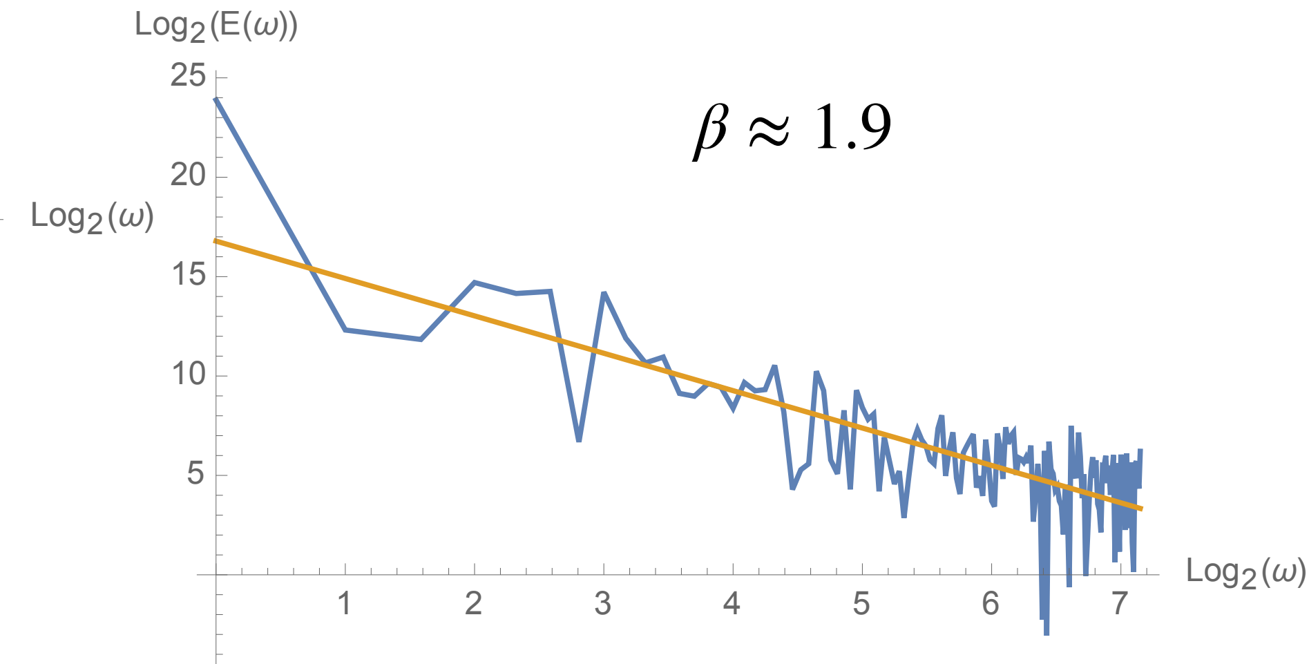
Vostok Dust
