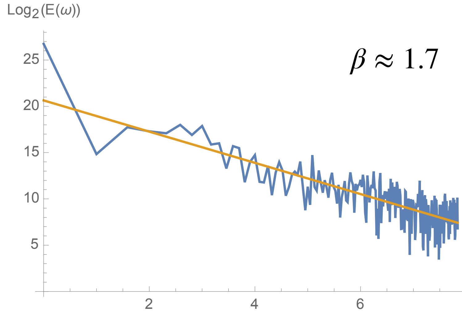
Vostok CH4
