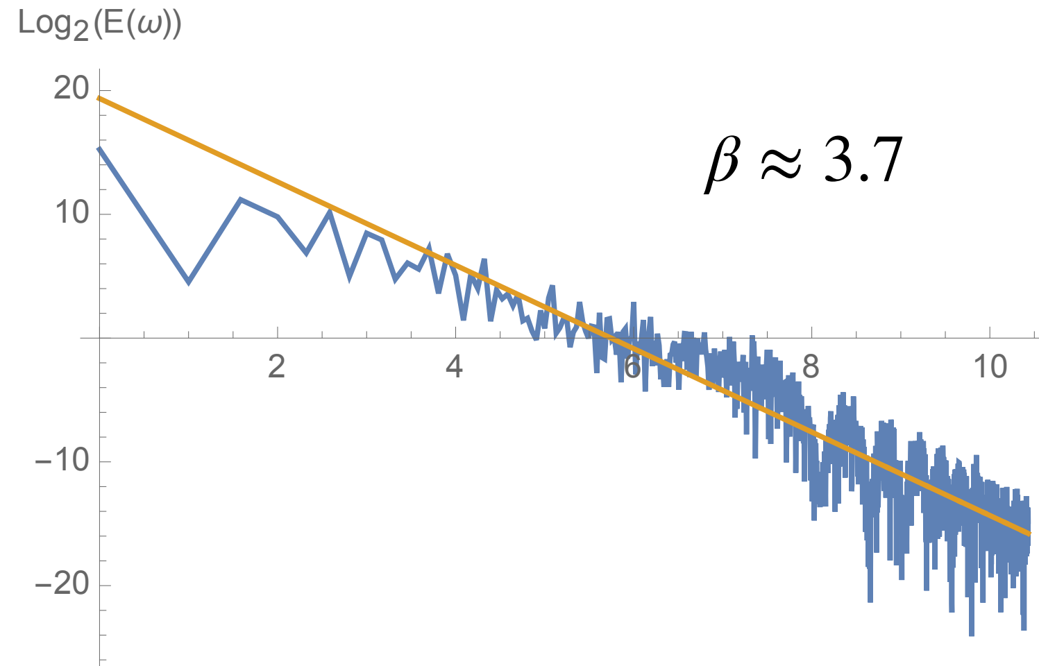
Vostok CH4
