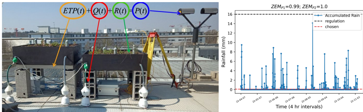
Figure 2. Prototypes expérimentaux mis en œuvre sur le toit de l'ENPC : lysimètre mesurant l'évapotranspiration en orange, débit en rouge, teneur en eau du substrat en vert et précipitation en bleu à l'aide d'un disdromètre
