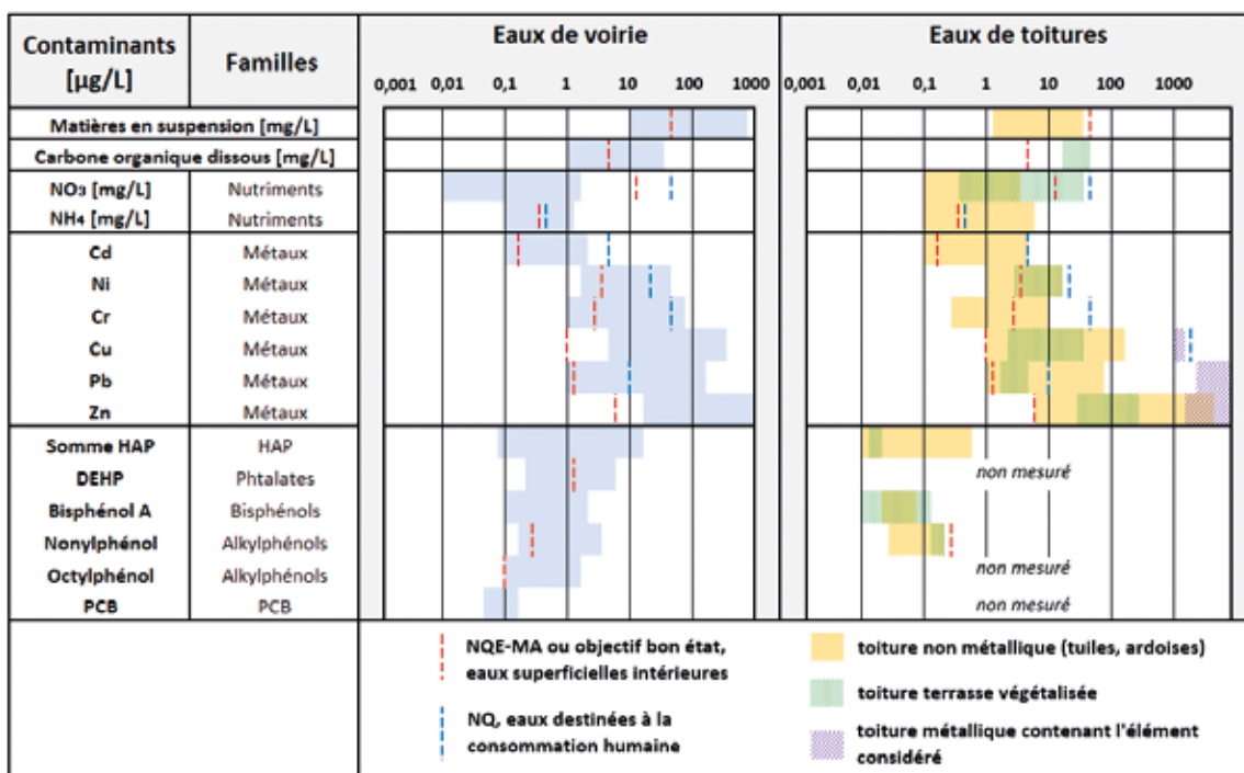
Figure 1.1 – Gamme de concentrations totales (dissoutes + particulaire) en différents contaminants dans les eaux de ruissellement de voiries et de toitures (adapté de Briand et al., 2018). Les plages de valeurs illustrent la variabilité inter-sites. NQ : Norme de Qualité ; NQE-MA : Norme de Qualité Environnementale (concentration moyenne annuelle à ne pas dépasser).
