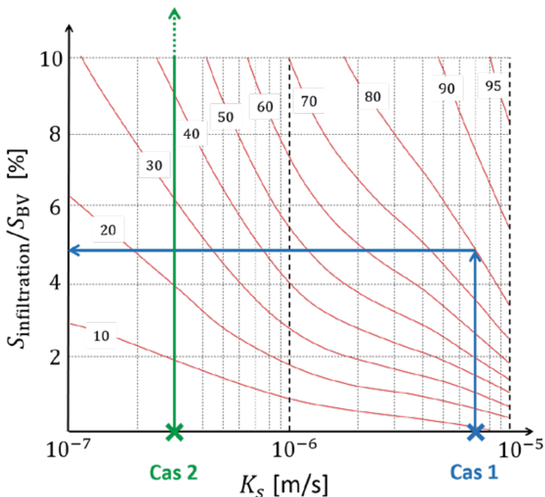
Figure 2.3 – Abaque présentant l'abattement (exprimé en %) pour les flux de contaminants à l'échelle pluriannuelle, en fonction de la perméabilité K_s et du ratio S_{infiltration}/S_{BV} , dans le cas d'une stratégie de régulation sans volume mort ( Q_{max} = 1 L/s/ha et h_p = 0 ).
