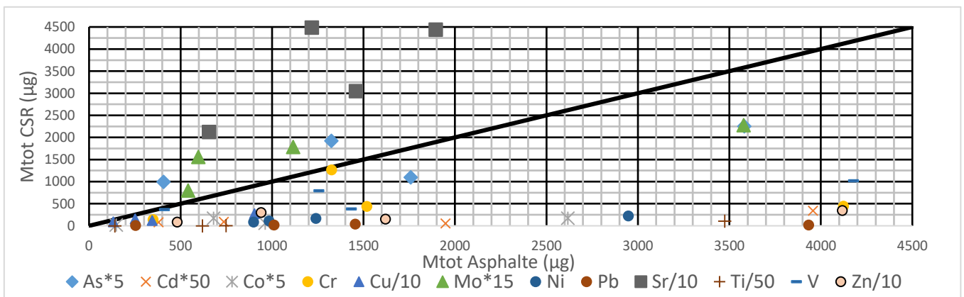
Figure 3 : Abattement en masse totale événementielle M_{tot} de différents métaux et métalloïde par la CSR comparées à celles produites sur la même surface par le parking asphalté sur 4 campagnes de prélèvement de novembre 2017 à mars 2018.
