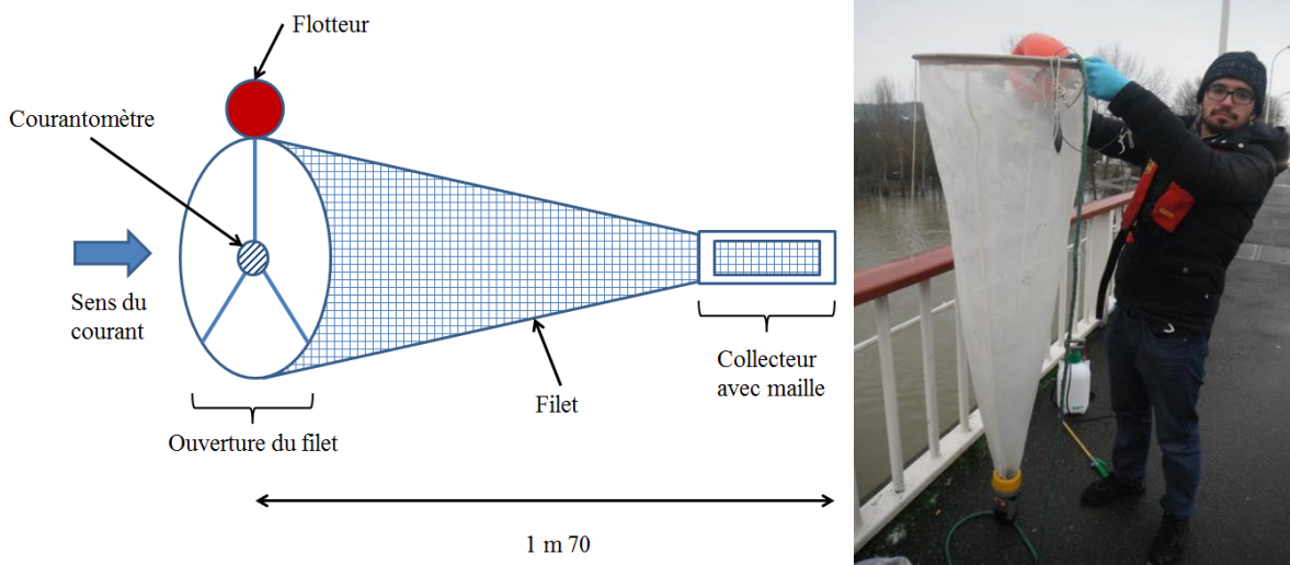
Figure 5 : Schéma et photographie du filet 330 \mu\text{m} (Photographie prise par R. Tramoy)
