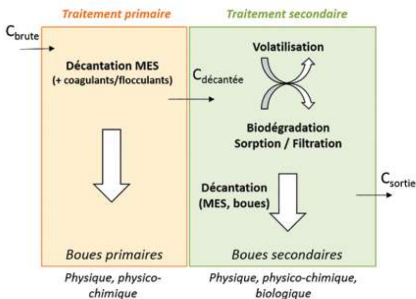
Figure 18 : Processus intervenant dans les différents traitements en STEU (filrière classique, modifiée d'après Scholes et al., 2008).
