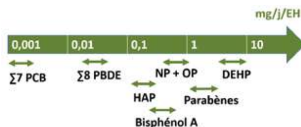
Figure 8 : Ordre de grandeur des flux unitaires de micropolluants organiques par jour et par équivalent habitant (EH) calculés sur l'année 2014 pour l'agglomération parisienne, NP : nonylphénols, OP : octylphénol.
