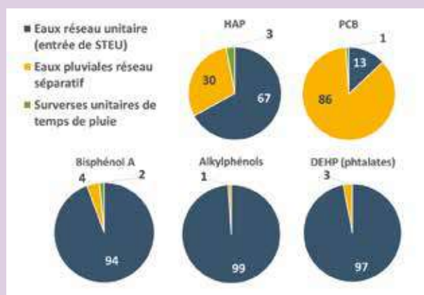
Figure 14 : Contribution relative des différentes eaux urbaines aux flux totaux annuels de micropolluants véhiculés dans les réseaux unitaire et séparatif de la zone SIAAP ( \Sigma 16 HAP, DEHP, AP : alkylphénols et éthoxylés), \Sigma 7 PCB) 15 (Briand et al. , 2016).
