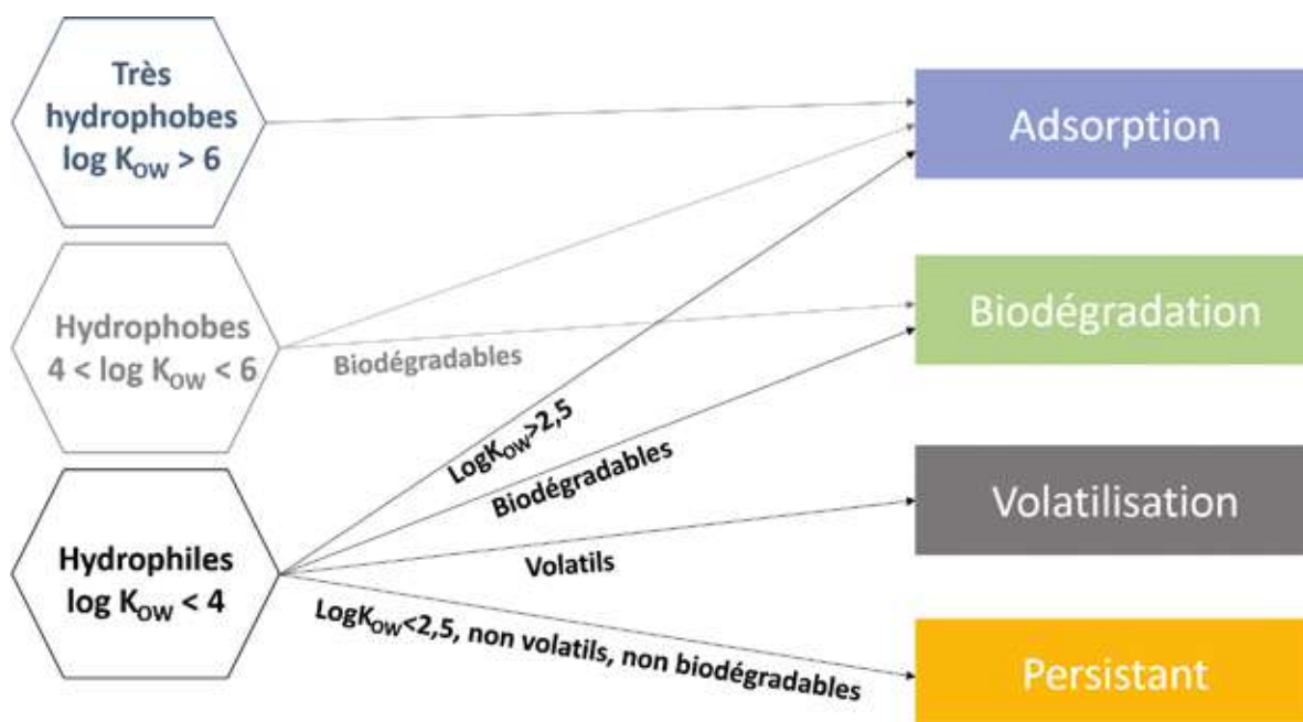
Figure 17 : Exemple de différents devenir de micropolluants en STEU en fonction des propriétés des molécules (modifiée d'après Mailler, 2015).
