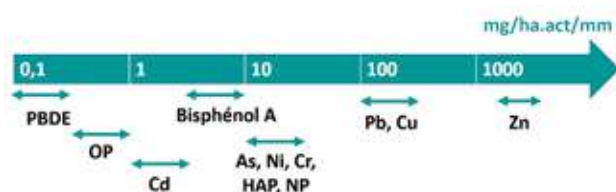
Figure 10 : Flux unitaires de micropolluants dans les eaux pluviales par hectare actif et par millimètre de pluie calculés pour trois bassins versants français (Chassieu, Pin Sec, Sucy, Hannouche et al., 2017). NP : nonylphénols, OP : octylphénol.
