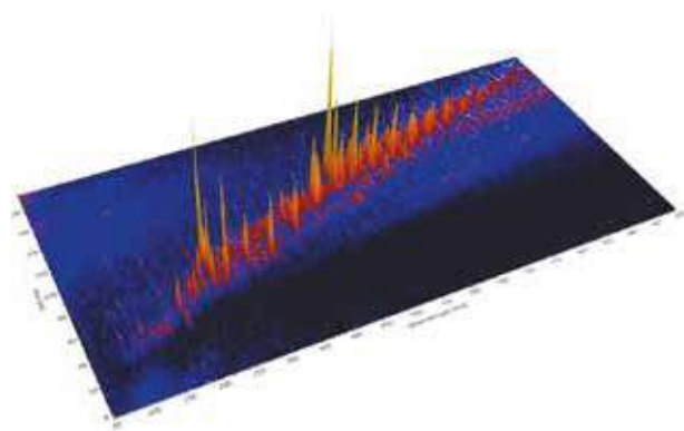
Figure 27 : Chromatogramme 3D d'un échantillon environnemental obtenu en spectrométrie de masse haute résolution (UPLC-QTOF). Masse (en abscisse) et temps de dérive (en ordonnée) des composés (source LEESU).
