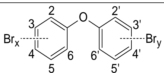
Figure 3. Formule générale des PBDE.
