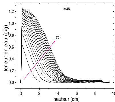
Figure 2: Distribution de teneur en eau le long de l'axe longitudinal, les profils sont présentés toutes les 4 heures
