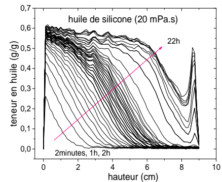
Figure 3: Distribution de teneur en huile de silicone le long de l'axe longitudinal : au début profils toutes les 2 minutes, puis toutes les heures et enfin toutes les 2 heures.
