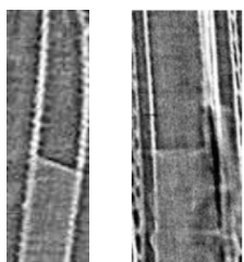
Fig. 3 : Interfaces eau/air planes observées dans des vaisseaux Fig. 4 : Interface eau/huile avec un angle de contact environ 20^\circ
