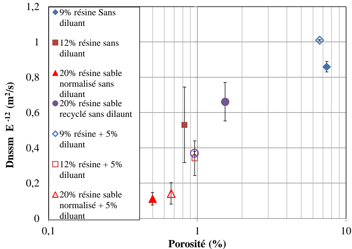
Evolution du coefficient de diffusion des ions chlorures en fonction de la porosité
