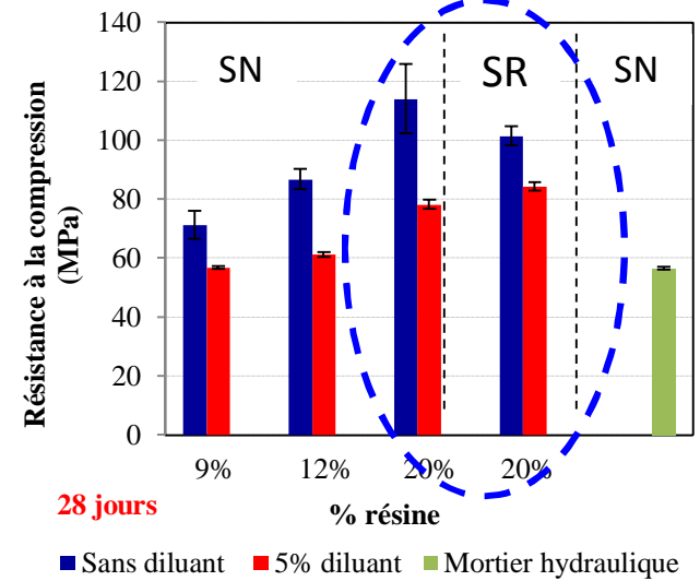
Evolution de la résistance à la compression en fonction du pourcentage de résine, du pourcentage du diluant et du type de sable.
