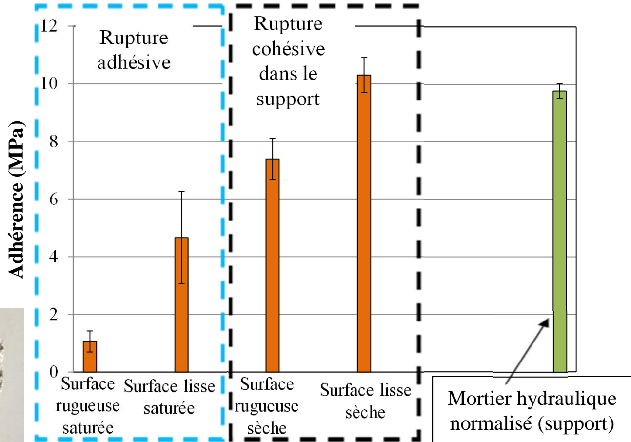
Adhèrence du mortier de réparation au mortier support et modes de rupture en fonction de l'état de surface
