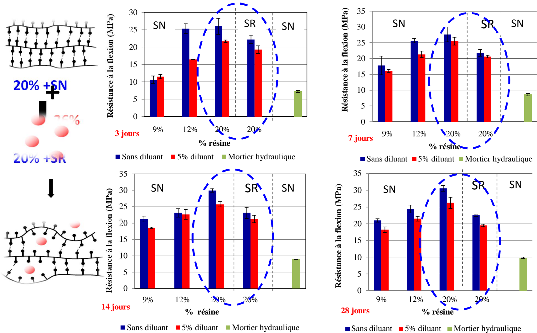
Evolution de la résistance à la flexion en fonction du pourcentage de résine, du pourcentage du diluant et du type de sable.
