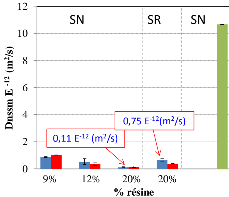
Diffusion des ions chlorures : NT Build 492
