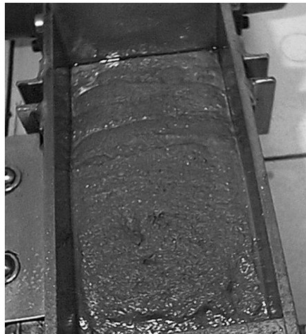
Figure 5 : Ecoulement du mortier dans un maniabilimètre ( E/C = 0,40 ; H/C = 0,7\% )
