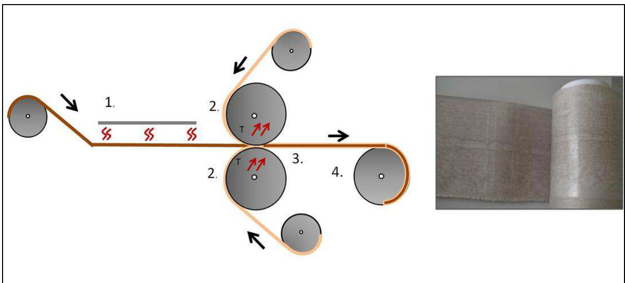
Figure 7: schéma de la production continue de preregs et une image du preregs enroulé
