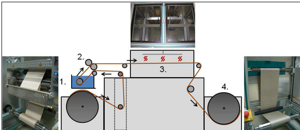
Figure 5: Schéma et images du procédé de revêtement continu du renfort pour l'amélioration de l'adhésion
