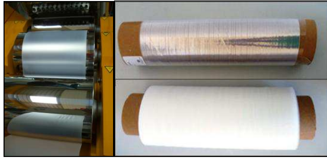
Figure 2: système à calandre (à gauche), Bio-ressourcés films Bio-PA (en haut à droite) et Bio-PE (en bas à droite)
