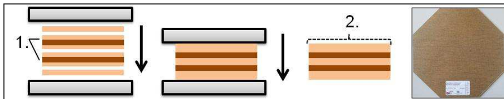
Figure 8: Formation d'un composite à plusieurs couches par moulage en compression
