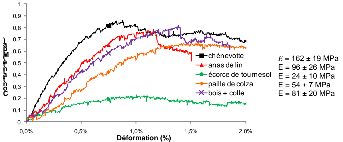
Figure 4 : Courbes de l'évolution de la contrainte en fonction de la déformation des matériaux élaborés lors d'essais de flexion trois points. La valeur ajoutée à côté de chaque légende est la moyenne du module d'élasticité obtenue après les cinq essais ainsi que l'écart-type résultant.
