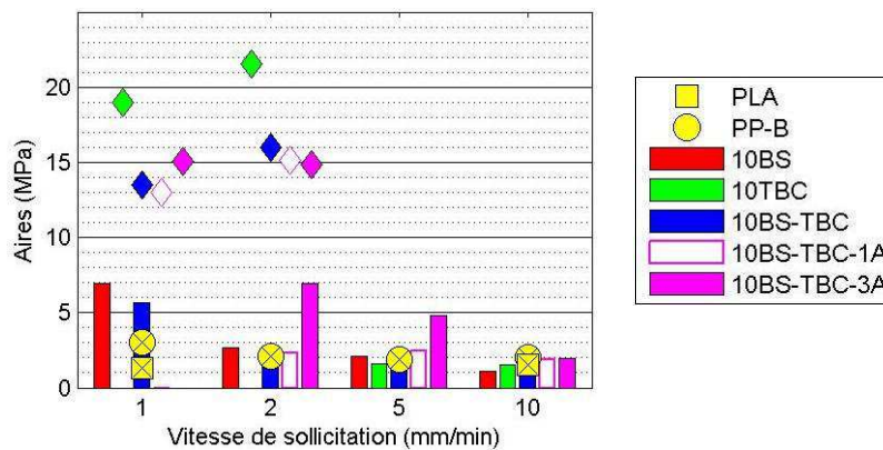
Figure 8 : aires sous les courbes de comportements nominaux (Eq. 3) (les losanges indiquent les valeurs moyennes atteintes pour des éprouvettes non rompues)
