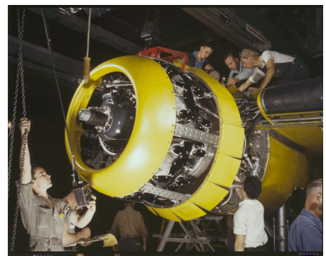
MONTAGE D'UN MOTEUR SUR UN FAIRFAX B-25 BOMBER, USINE DE NORTH AMERICAN AVIATION, INC., INGLEWOOD, CALIFORNIE.
