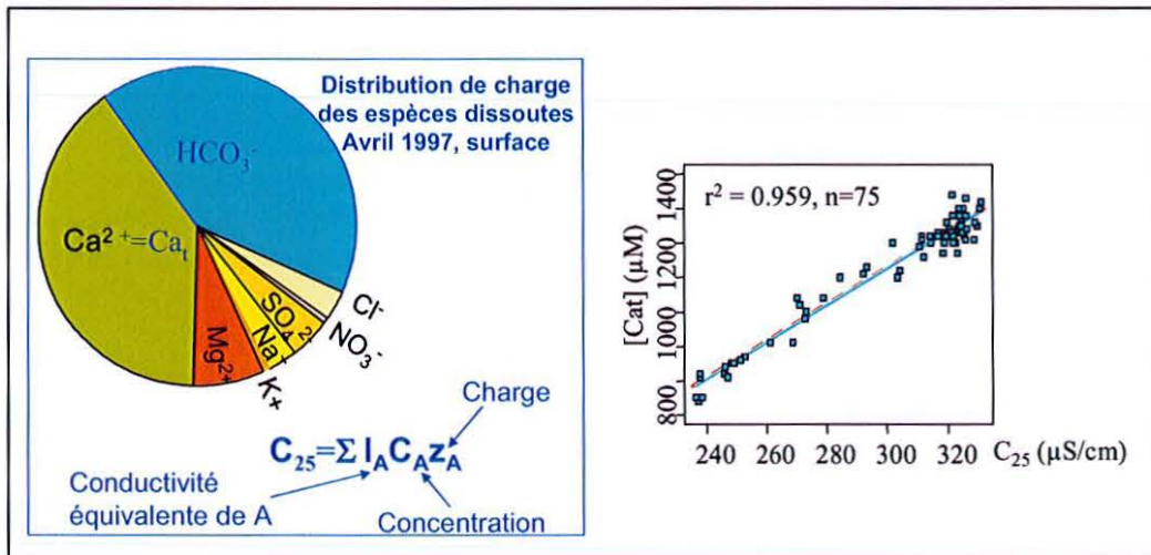
Figure 4. Relation entre Calcium dissous et Conductivité spécifique dans l'épilimnion du lac du Bourget (d'après Groleau et al. , 2000).
