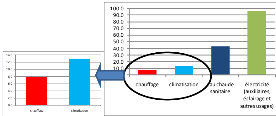
Figure 2 : consommation par postes en kWh/m 2 par an pour le projet Ecocatif en bois (Ecocatif, 2009)
