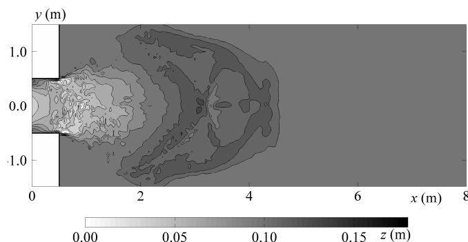
Figure 16. Final bed topography for Case 2 from IST
