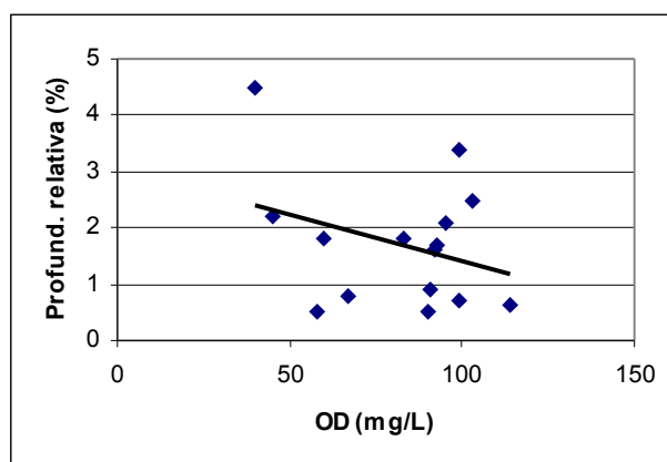
Figura 5 - Relação entre Oxigênio Dissolvido na superfície e Profundidade Relativa
