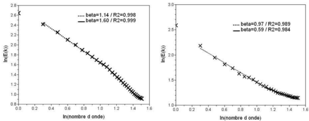
Figure 6 : Moyenne d'ensemble des spectres en analyse temporelle : Més0-NH (à droite) et radar (à gauche)
