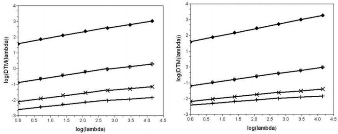
Figure 7 : DTM ( q=1.5 , \eta=0.66 ; 1 ; 1.52 ; 2.31) en fonction de la résolution en graphique log-log pour l'analyse temporelle en moyenne d'ensemble. (à gauche) Simulation Més0-NH (à droite) Données radar. Les coefficients de régression linéaire R^2 pour les grandes échelles, pour les petites échelles et sans prendre en compte de rupture valent respectivement 0.99, 0.99 et 0.98 pour les données Més0-NH et 0.99, 0.99 et 0.99 pour les données radar.
