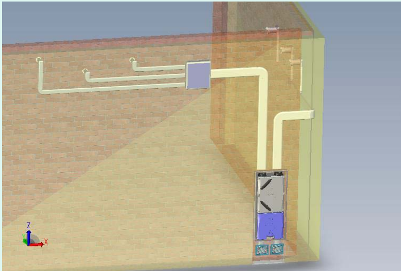
VMC Double Flux intégrée à l'ITE Fondation Bâtiment Energie, Projet MITECH
