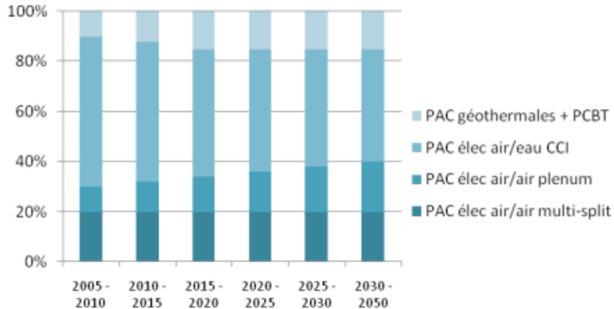
PAC en réhabilitation MI
